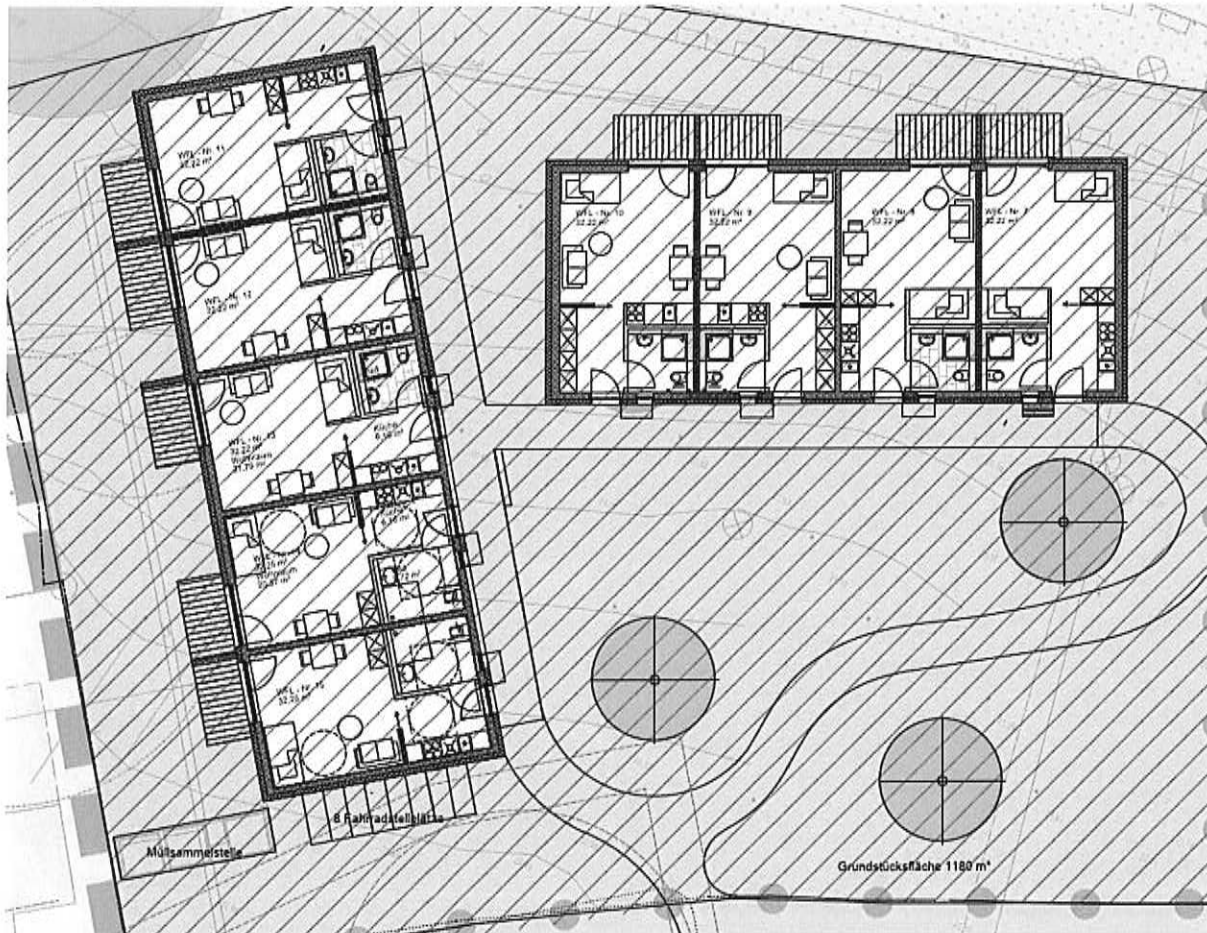
Abbildung 6 - Grundriss OG, Lorenzen - Silbernagel Architekturbüro
